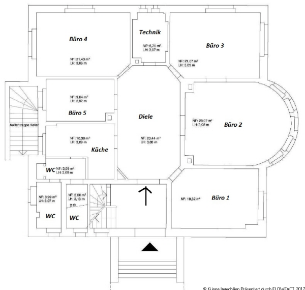
Grundriss
